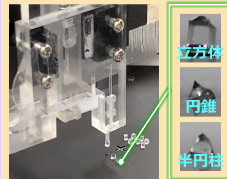
液架橋カグリッパ
